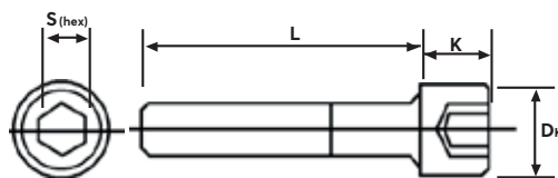
Dimensions to BS EN ISO 4762 DIN 912
